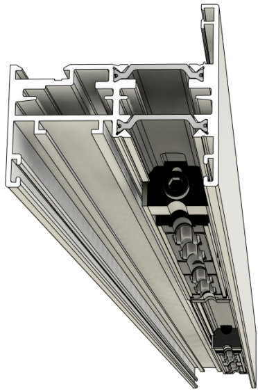
2 Carrelli portata singola anta = 500 KG
