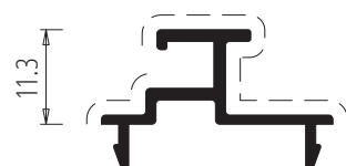
vz SM008 200 gr/m (scatta in vuoto 24 mm)
