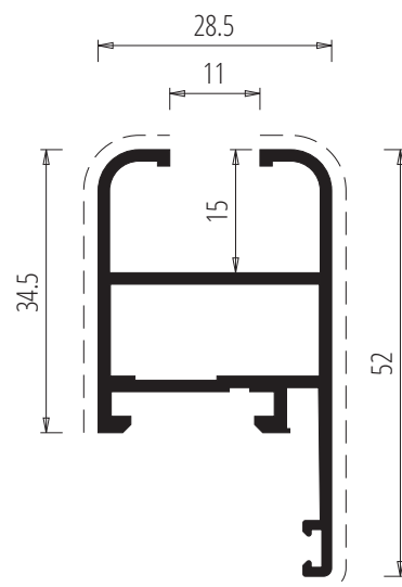
vz SM003 643 gr/m
