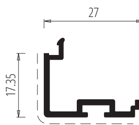
vz SM012 243 gr/m
