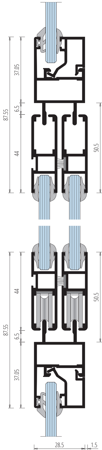
SEZIONE VERTICALE CON PROFILI SCORREVOLI
