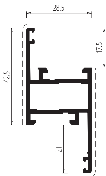
vz SM013 689 gr/m
