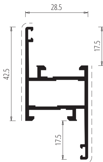
vz SM002 674 gr/m
