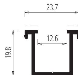
vz 0786 258 gr/m (scatta in vuoto 24 mm)
