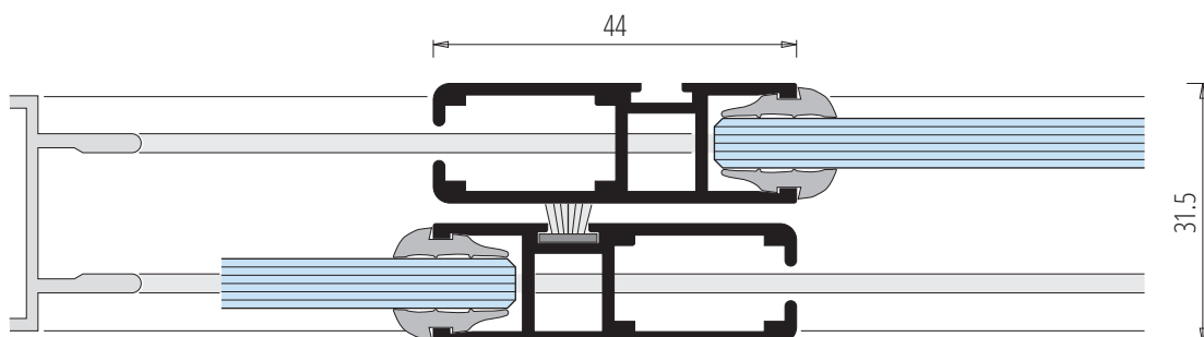
SEZIONE CENTRALE CON ANTE SCORREVOLI
