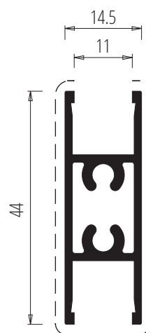
vz SM022 537 gr/m
