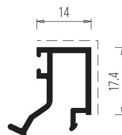
vz SM009 258 gr/m
