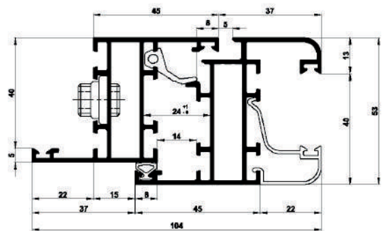
nodo laterale
