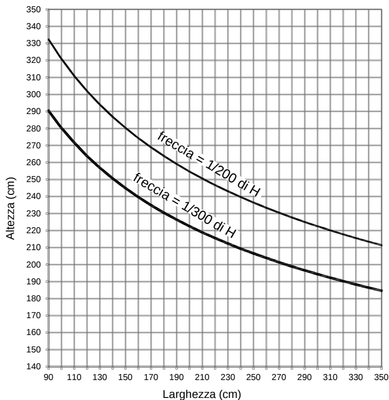
CARICO DEL VENTO 600 Pascal
