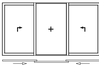
FINESTRA 2 ANTE SCORREVOLI ESTERNE FISSO CENTRALE
