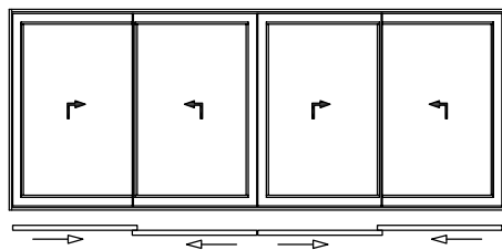
FINESTRA 4 ANTE CON NODI INTERMEDI 50mm
