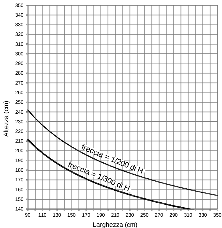
CARICO DEL VENTO 1200 Pascal
