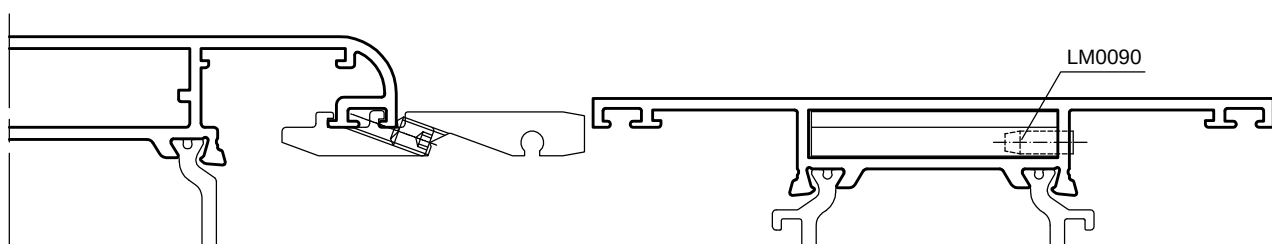
APPLICAZIONE SU ANTE
