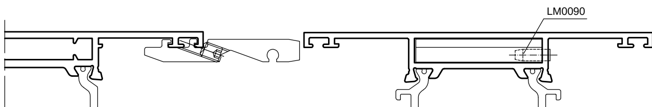
APPLICAZIONE SU ANTE COMPLANARI
