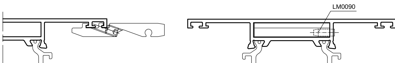
APPLICAZIONE SU TELAI
